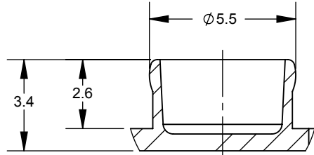
DETAIL B SCALE: 5 : 1 TYP
