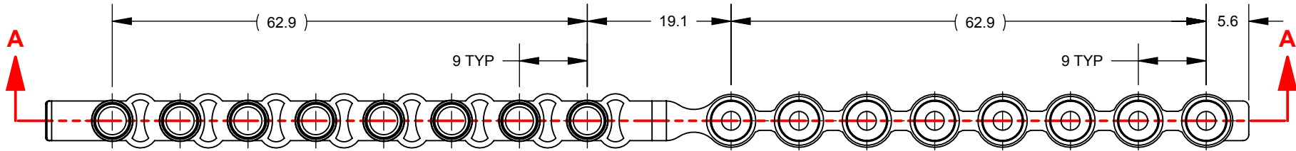
DETAIL C SCALE: 2.2 : 1 TYP
